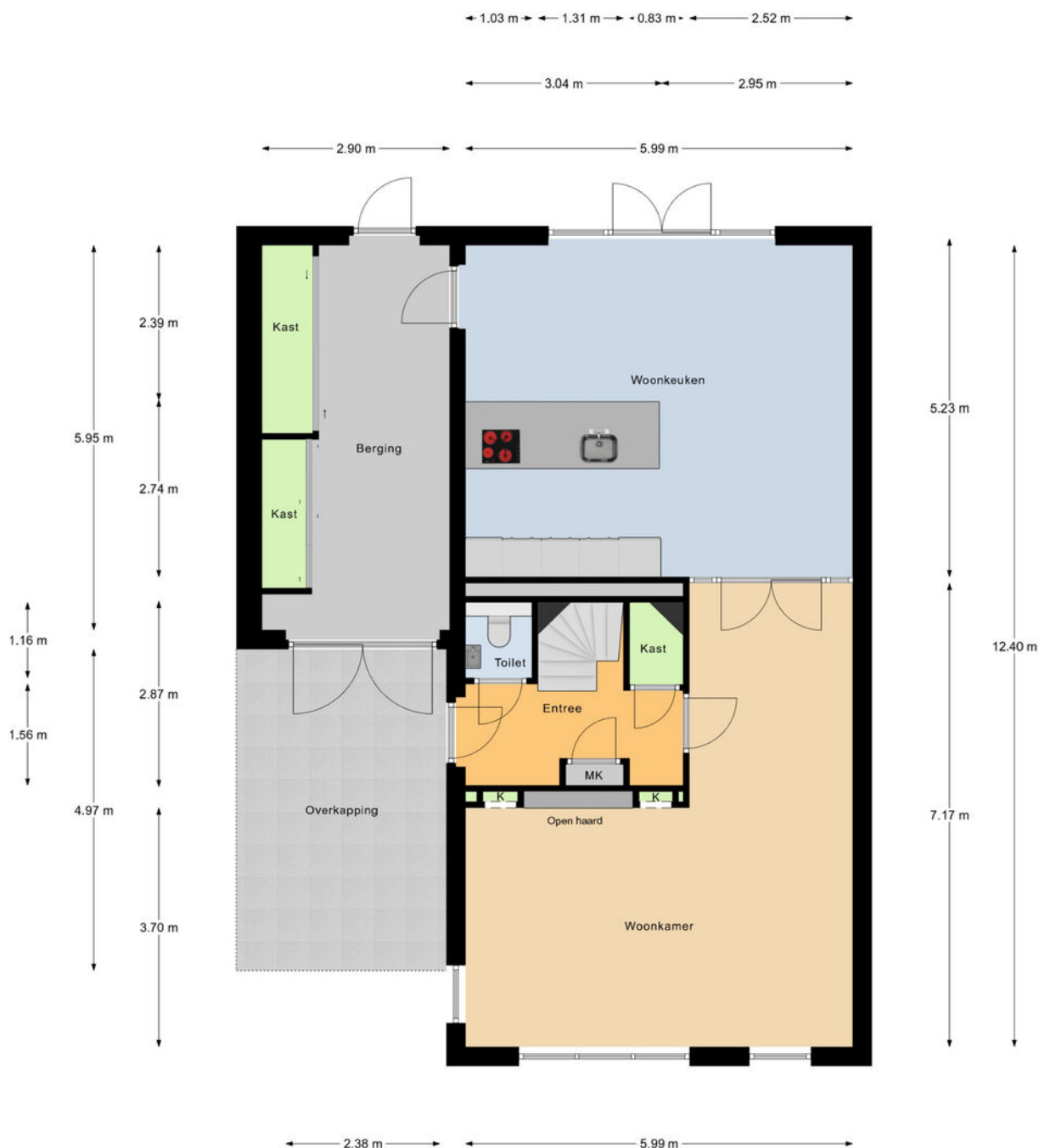
Begane Grond
